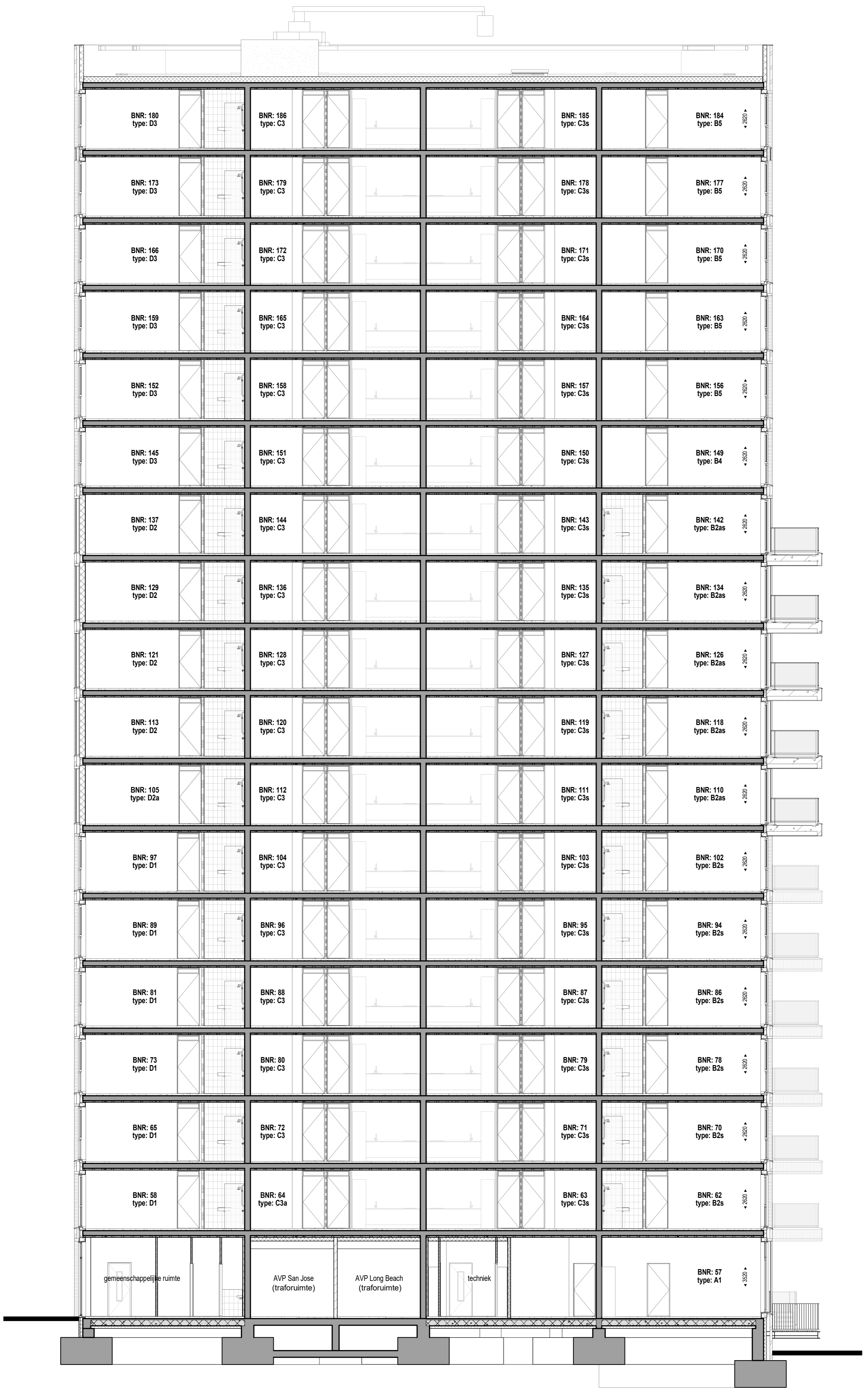
Doorsnede CB
