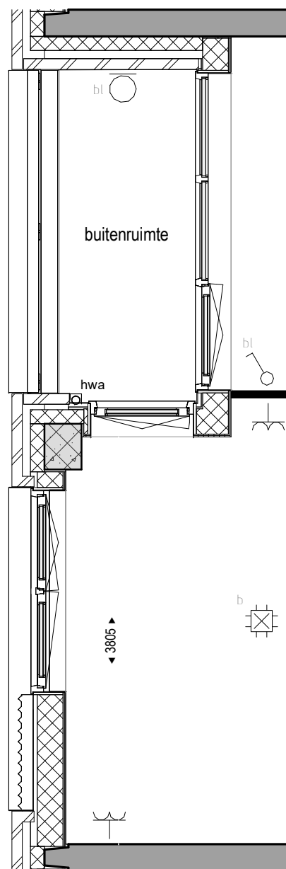
Gevelfragment verdieping 7 t/m 11 (Bouwnummers: 112, 120, 128, 136 en 144)
