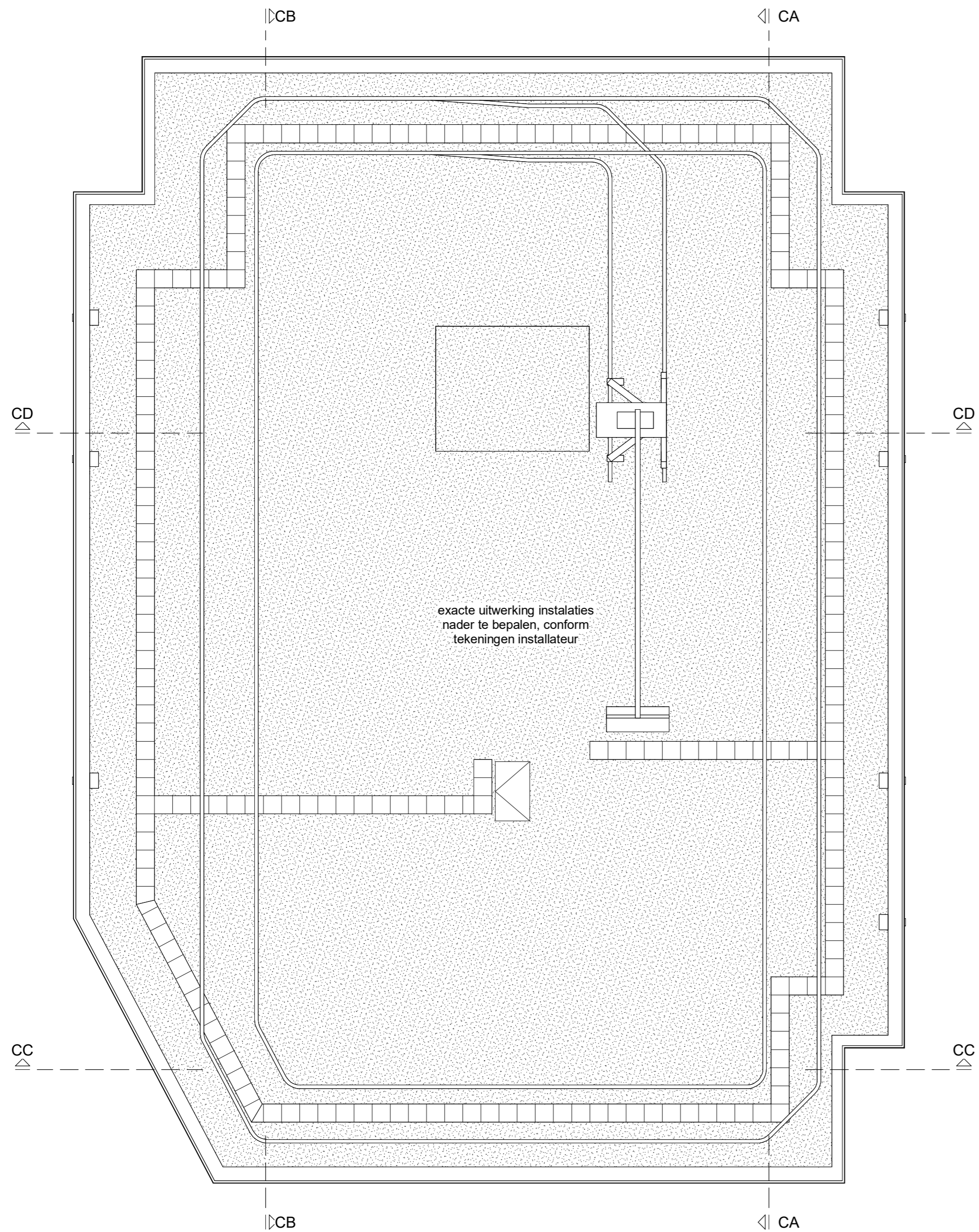
Dakaanzicht
