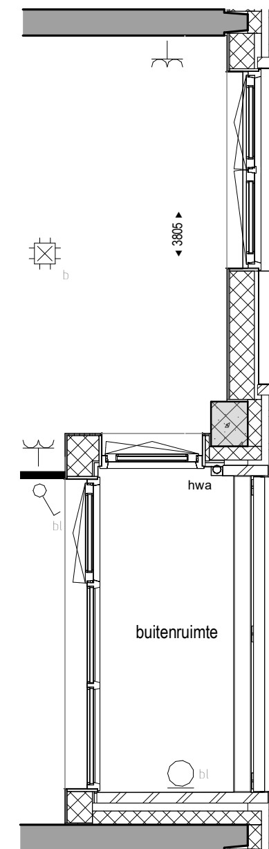
Gevelfragment verdieping 7 t/m 11 (Bouwnummers: 108, 116, 124, 132 en 140)
