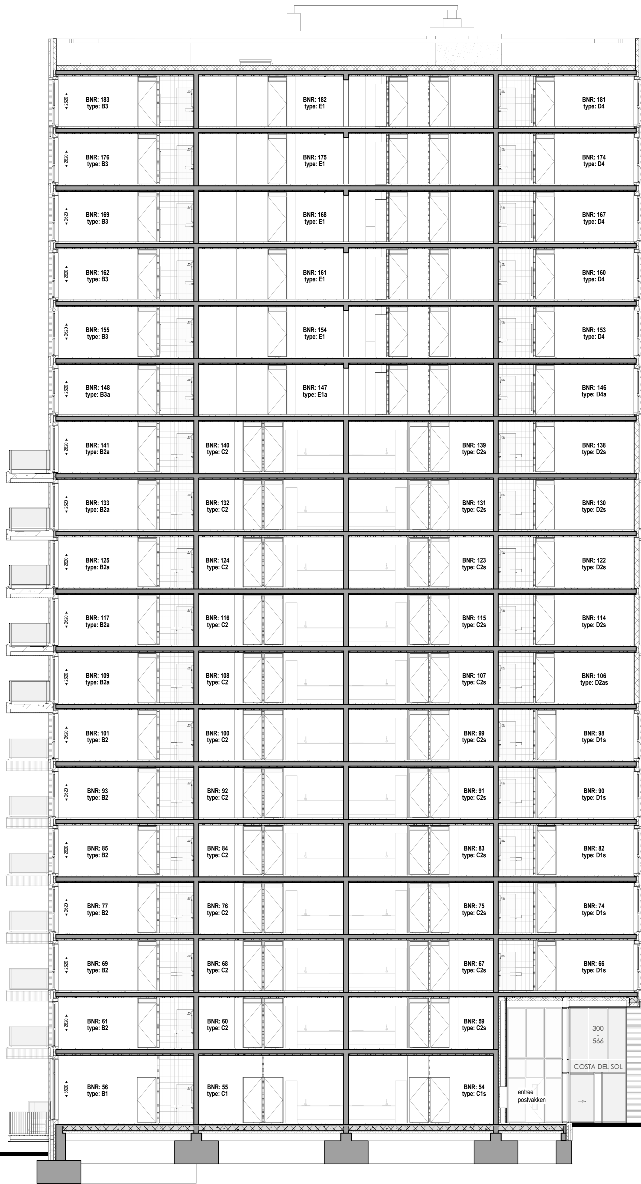
Doorsnede CA
