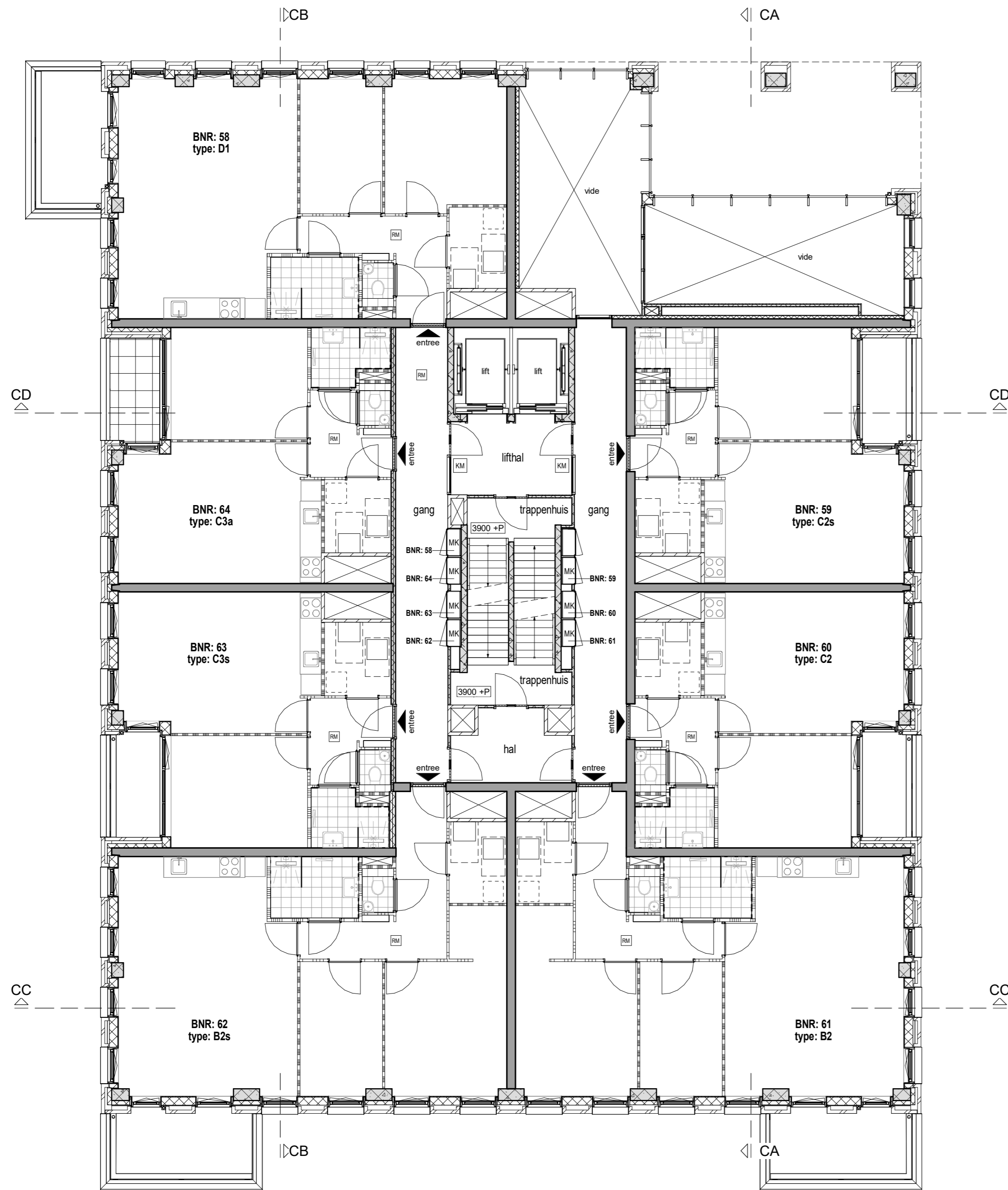
Verdieping 1
