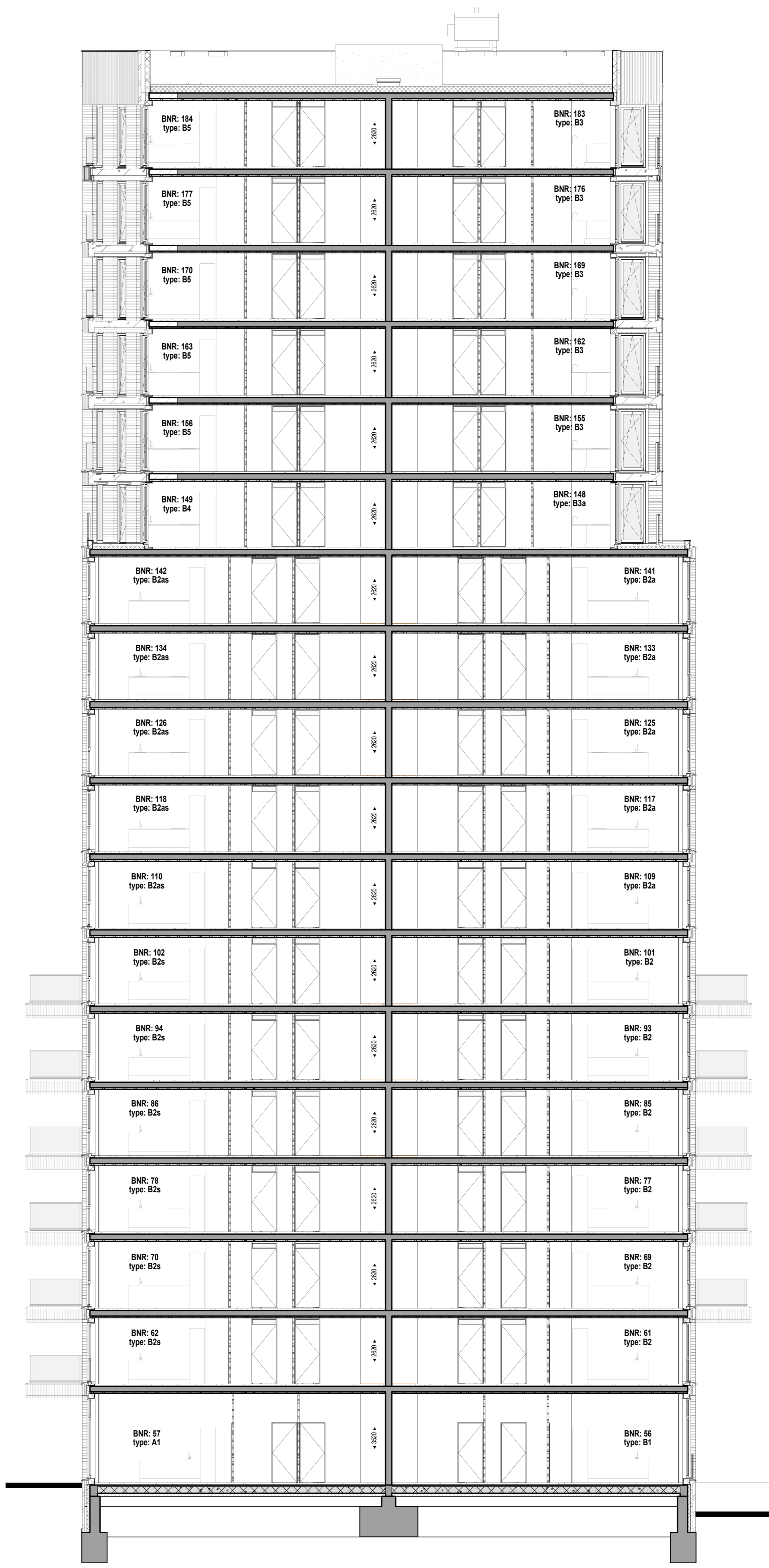
Doorsnede CC
