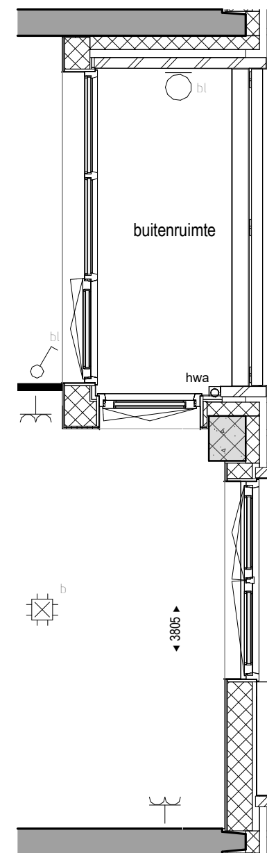
Gevelfragment verdieping 7 t/m 11 (Bouwnummers: 107, 115, 123, 131 en 139)
