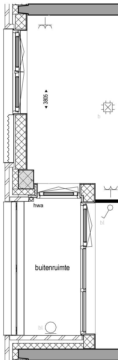
Gevelfragment verdieping 7 t/m 11 (Bouwnummers: 111, 119, 127, 135 en 143)
